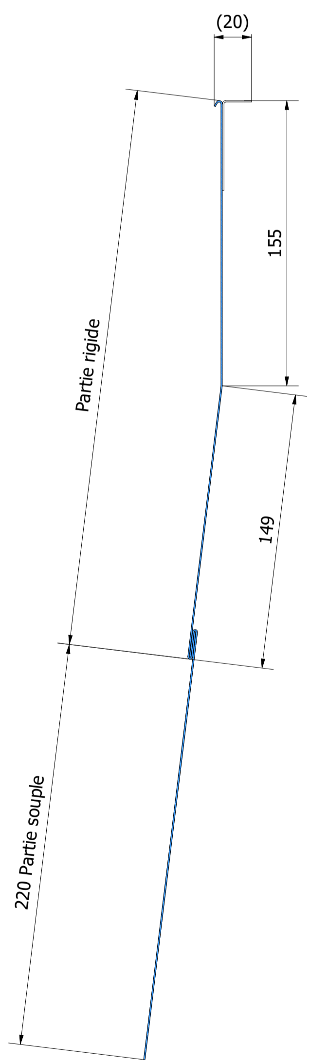
A-A ( 1 : 2 )
